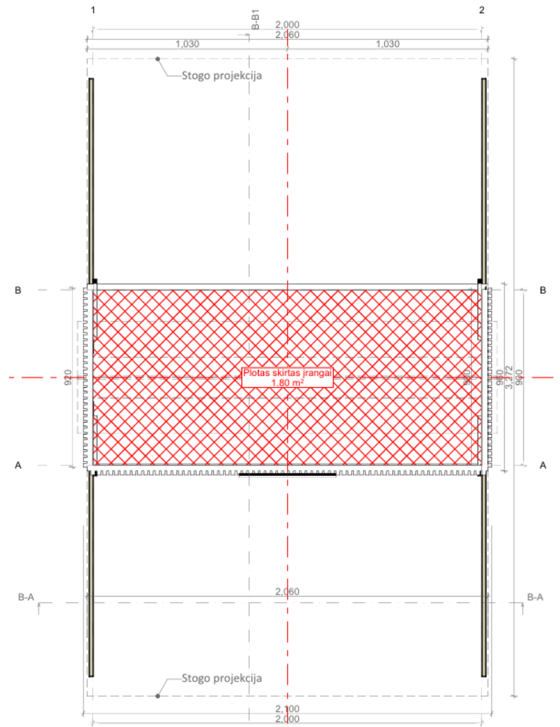
AUKŠTO PLANAS 1:20
