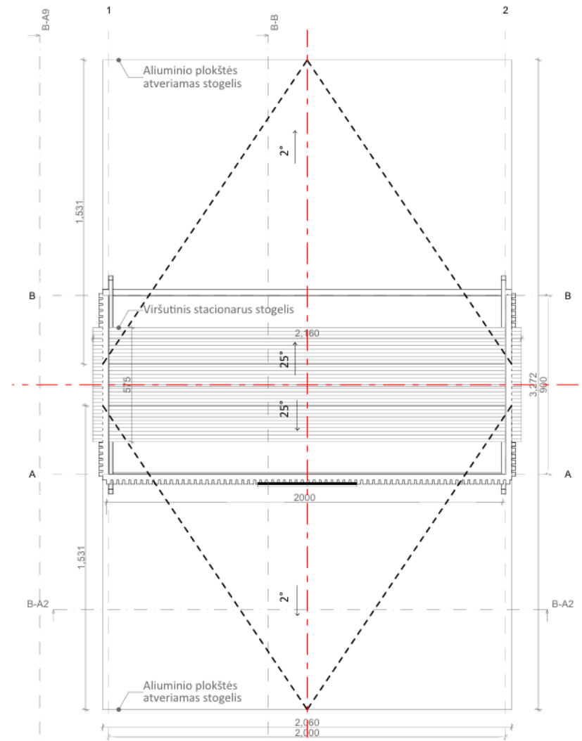
STOGO PLANAS 1:20
