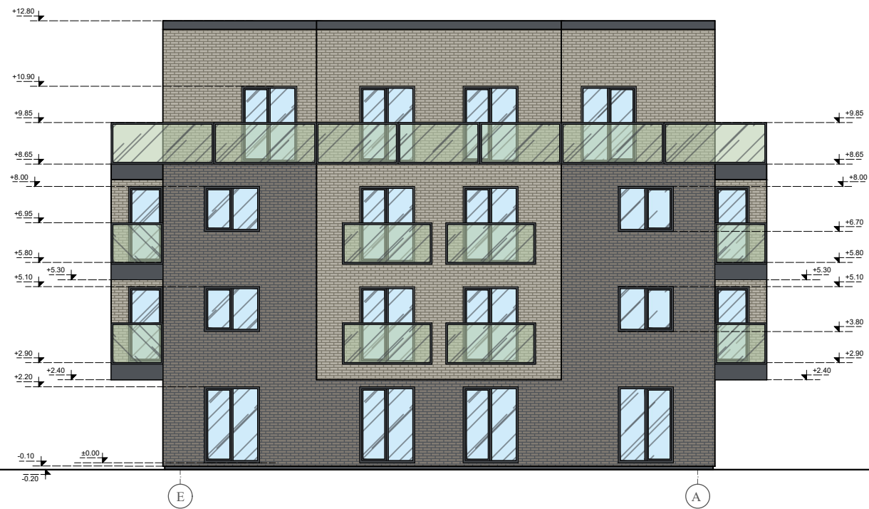
VAKARINIS FASADAS E-A 1:100
