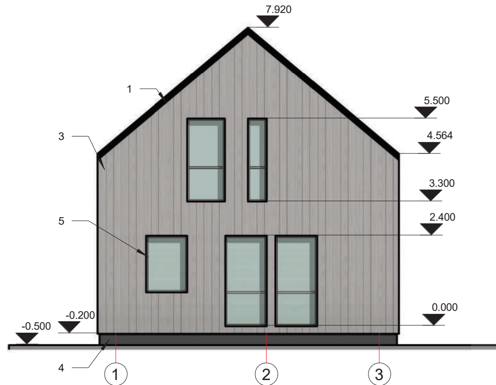
FASADAS TARP AŠIŲ 1-3 M1:100
