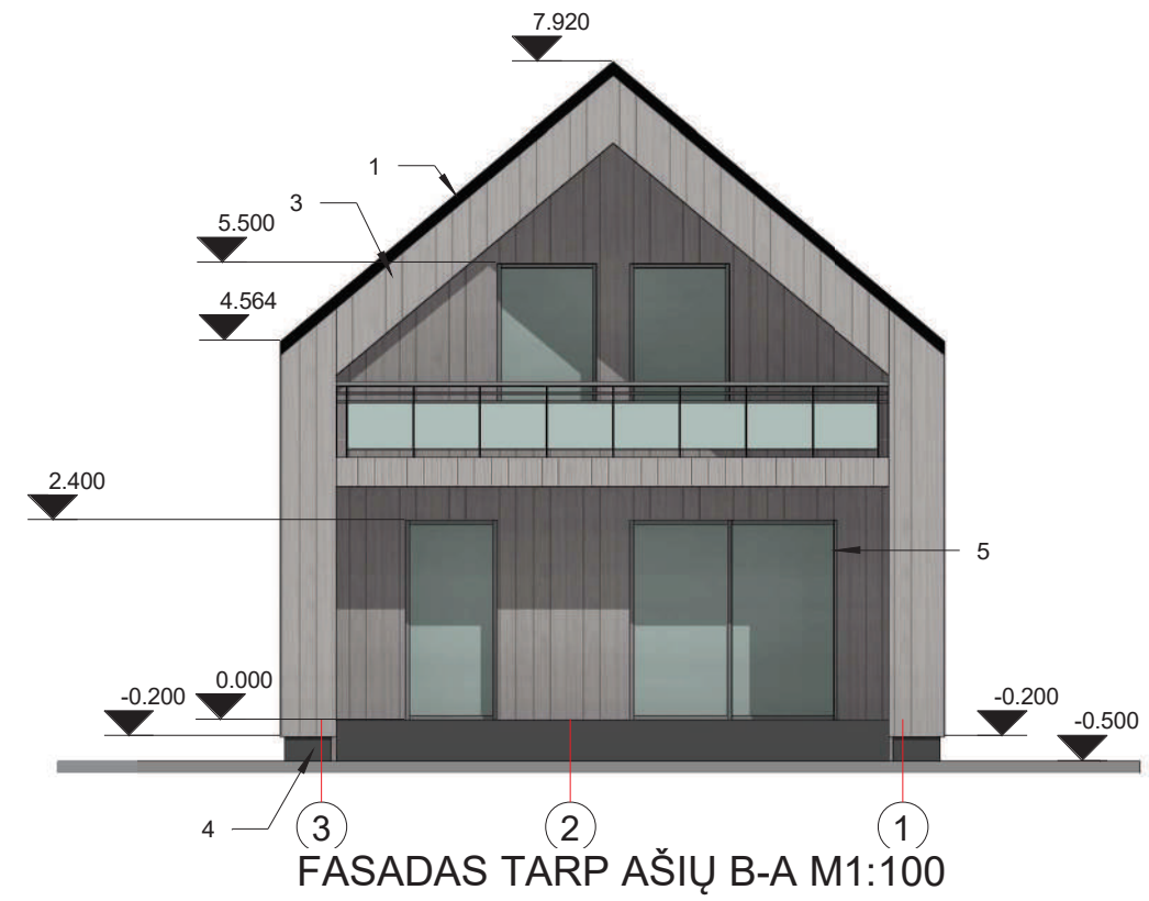
FASADAS TARP AŠIŲ 3-1 M1:100
