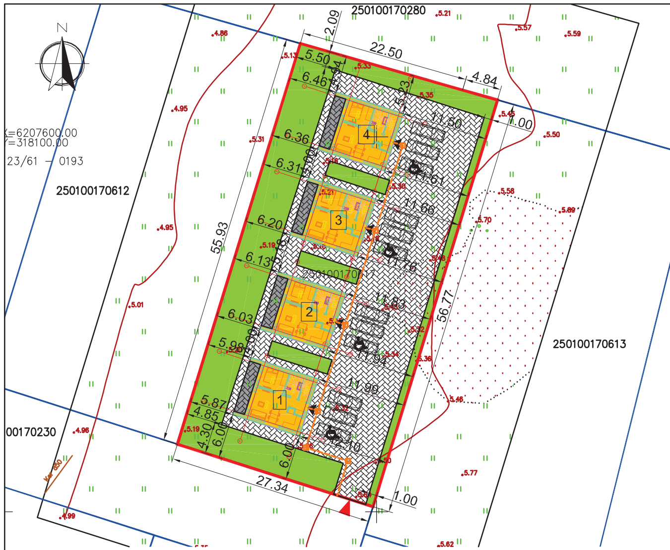
SITUACIJOS SCHEMA
