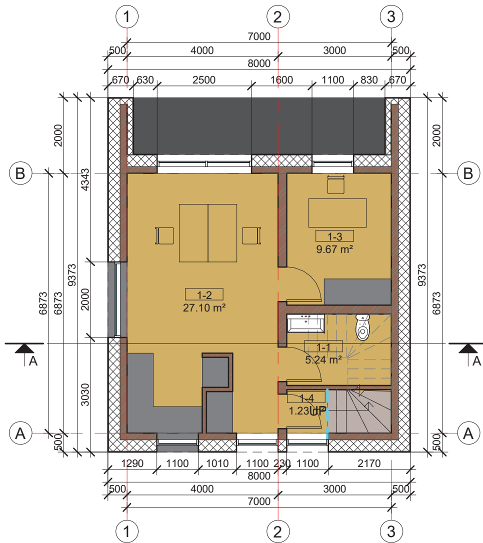
PIRMO AUKŠTO PLANAS M1:100
