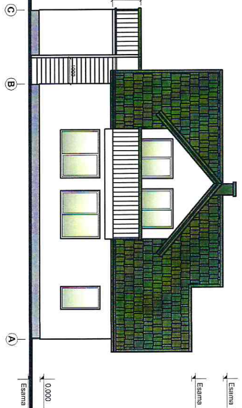
FASADAS TARP AŠIŲ C - A M 1:100
