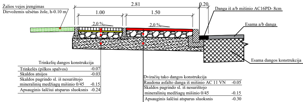
Pjūvis 1-1
